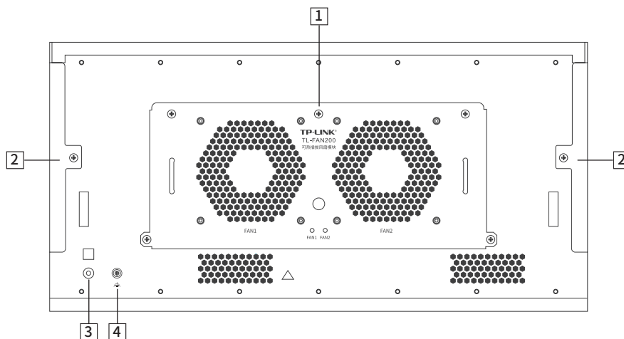
图1-5 TL-S7803机框结构示意图(背面)
