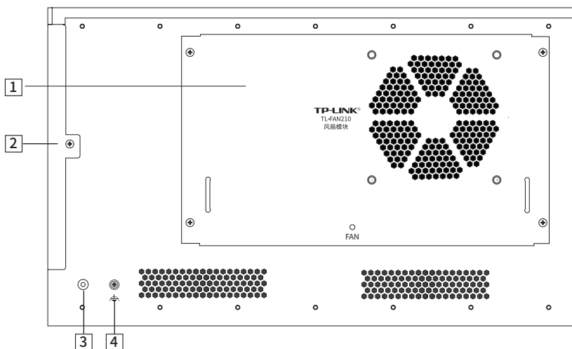
图1-9 TL-S7903机框结构示意图(背面)
