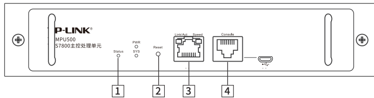
图1-11 TL-MPU500结构示意图
