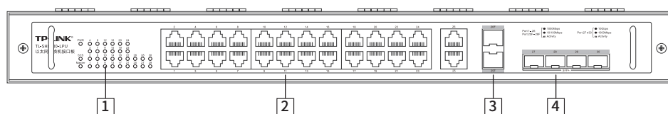
图1-15 TL-SH8430-LPU结构示意图
