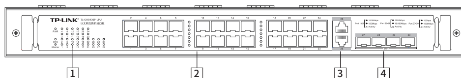
图1-19 TL-SH8430F-LPU结构示意图
