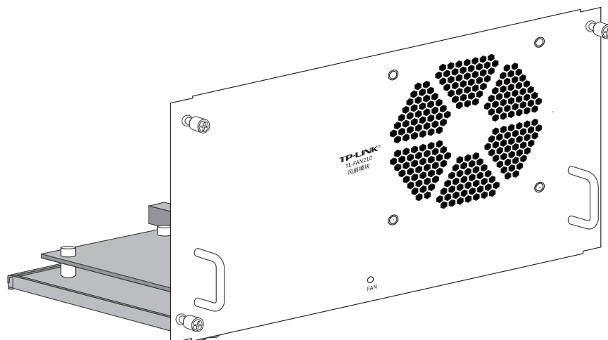
图1-28 TL-FAN210风扇模块外观
