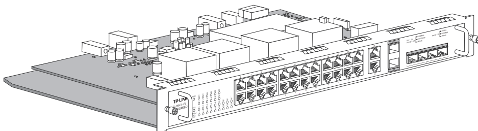
图1-14 TL-SH8430-LPU业务板外观
