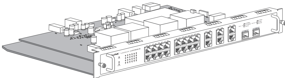
图1-12 TL-SH7224-LPU业务板外观
