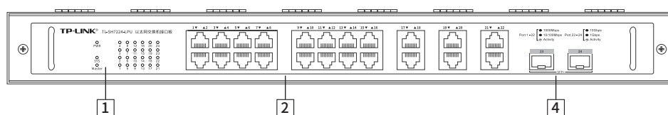
图1-13 TL-SH7224-LPU结构示意图
