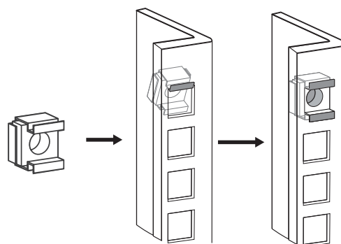
图2-3 浮动螺母安装示意图
